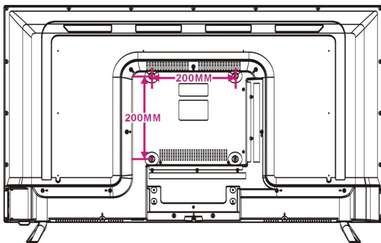
Televizoriaus nugarėlė
