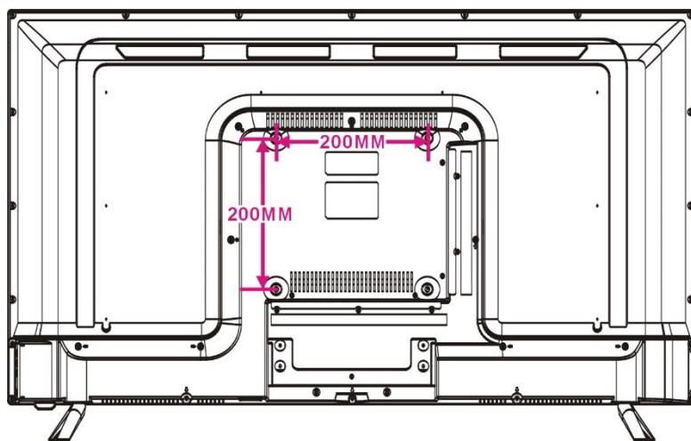
Televizora aizmugure
